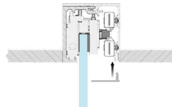
Deckenbündige Montage
