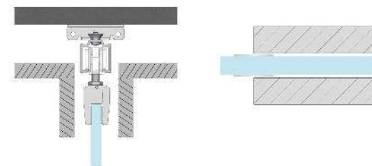
Deckenbündige Montage
